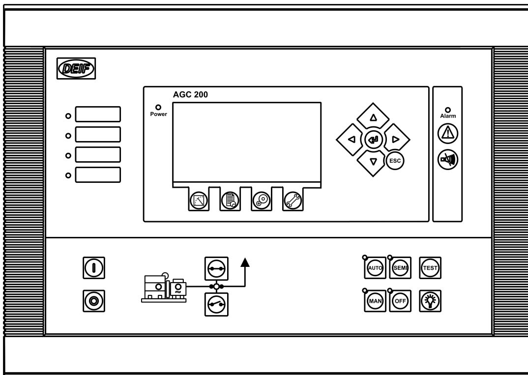
Лицевая панель генераторного контроллера AGC 222
